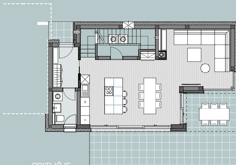
PRITLIČJE
